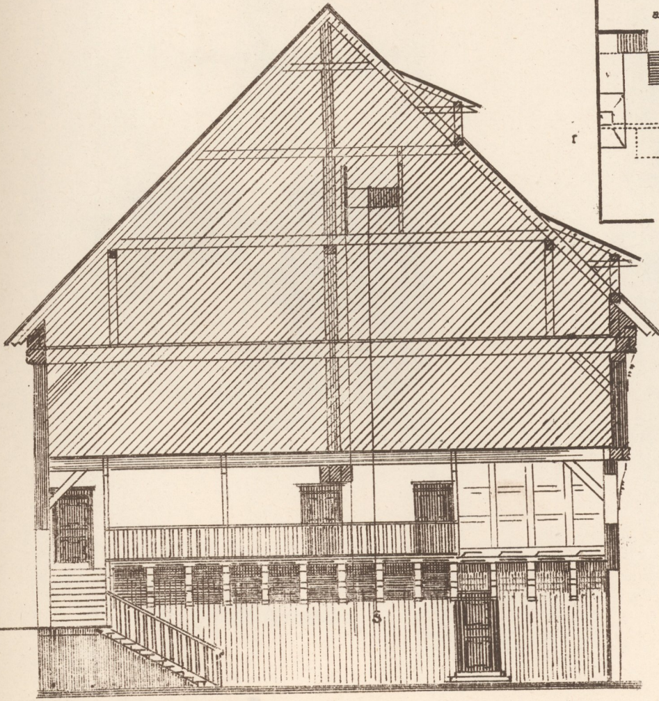
Querschnitt nach ab des Grundrisses.
