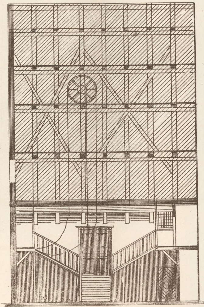
Längenschnitt nach rd des Grundrisses.
