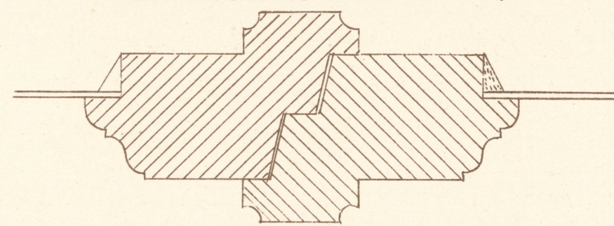
EINFACHES FENSTER.
