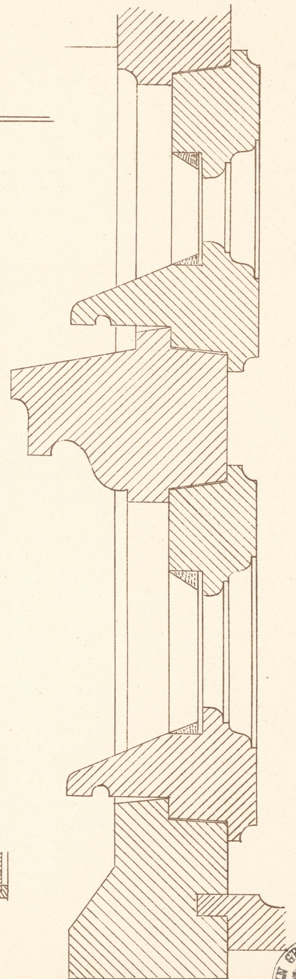
EINFACHES FENSTER.
