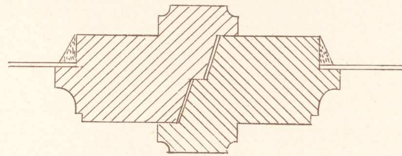
DOPPELFENSTER.
