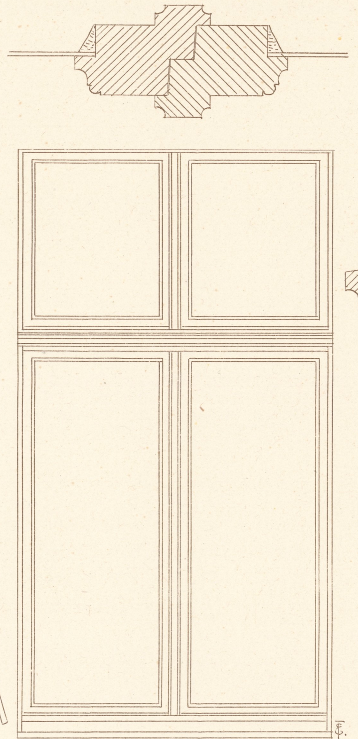
FENSTER MIT ROLLADENVERSCHLUSS.
