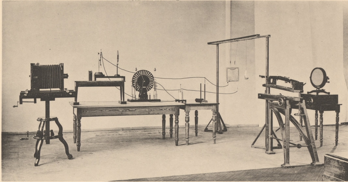
Versuchseinrichtung für die Mach'sche Funkenphotographie.
