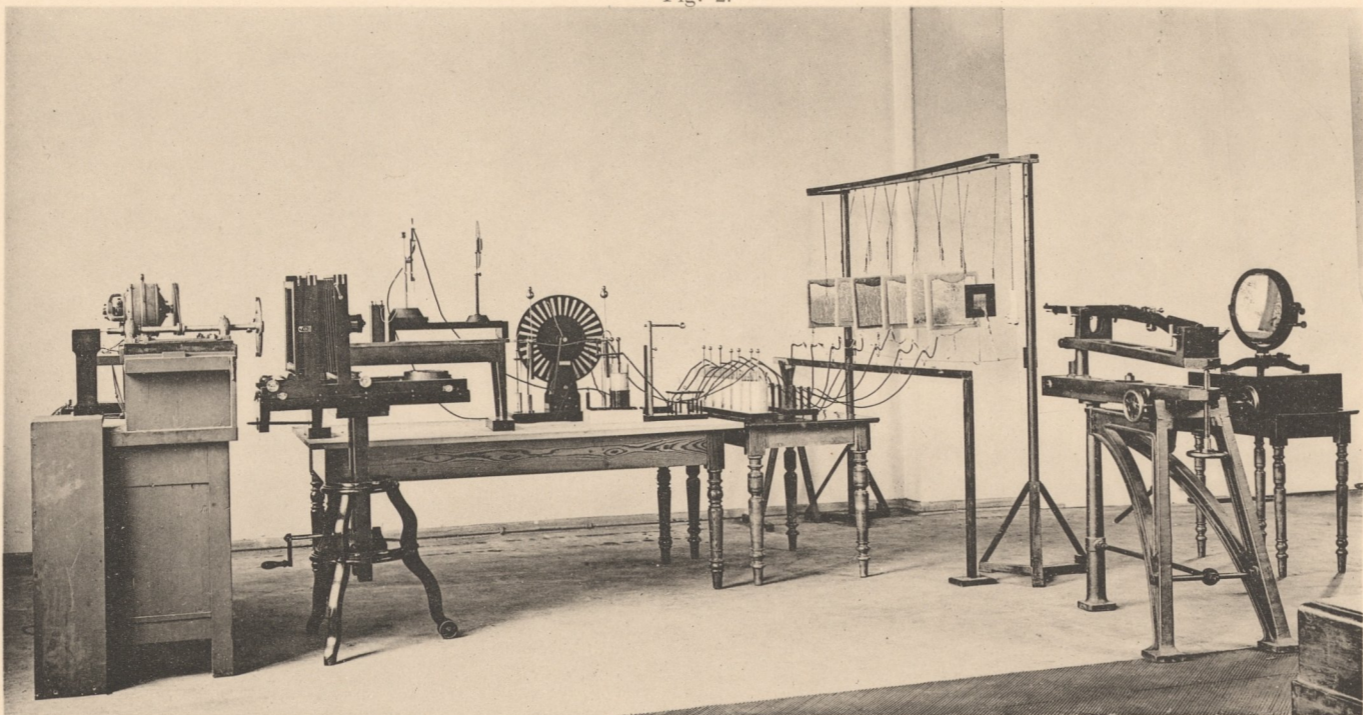
Versuchseinrichtung für die Mehrfachfunkenphotographie.
