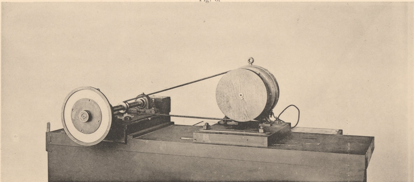
Rotierende Aufnahmescheibe für die Mehrfachfunkenphotographie.
