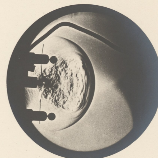
Geschoss beginnt aus dem Lauf auszutreten.
