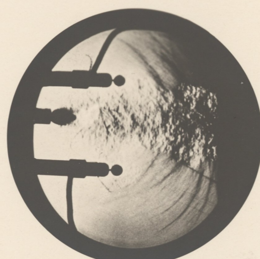
Geschoss im Begriff den Lauf zu verlassen.
