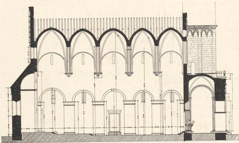
Längenschnitt.
