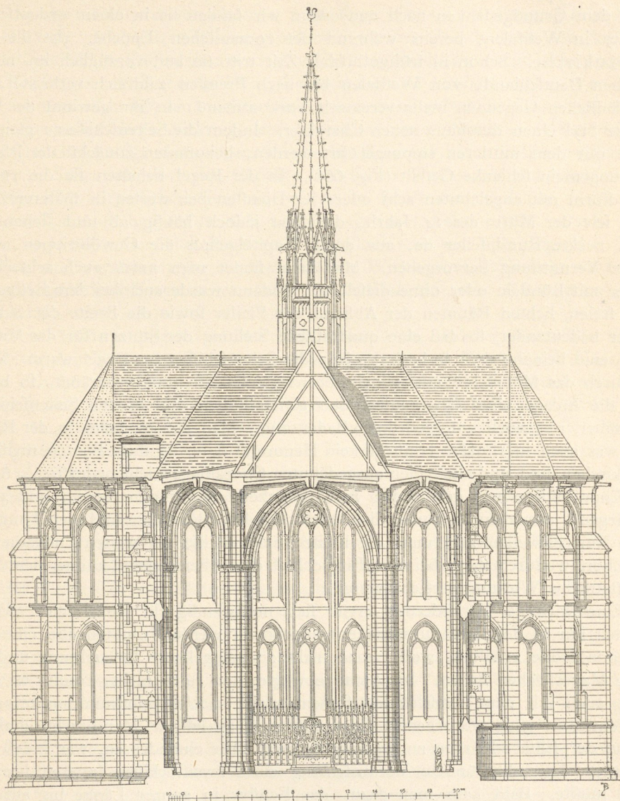
Fig. 660. St. Elisabethkirche zu Marburg. Querschnitt. (Nach Moller.)
