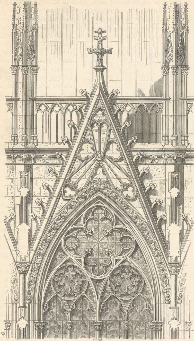
Fig. 587. Wimperge vom Kölner Dome. (Baldinger.)
