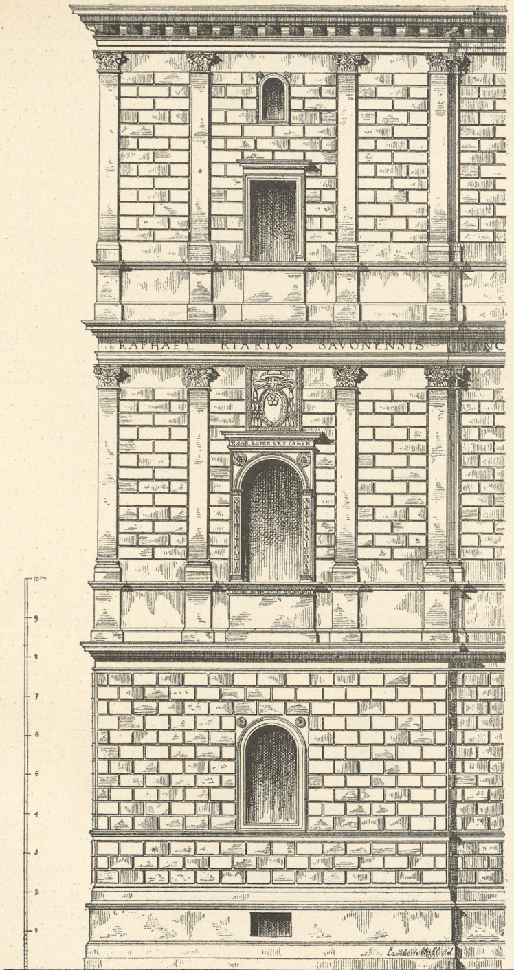
Fig. 832. Von der Cancelleria zu Rom. (Lambert u. Stahl.)
