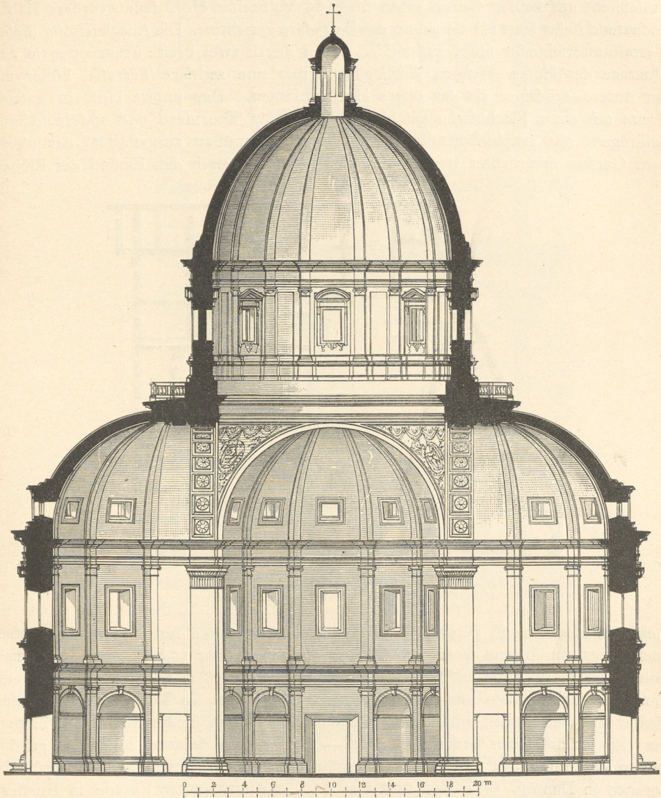
Fig. 830. Mad. della Consolazione in Todi. (Laspeyres.)
