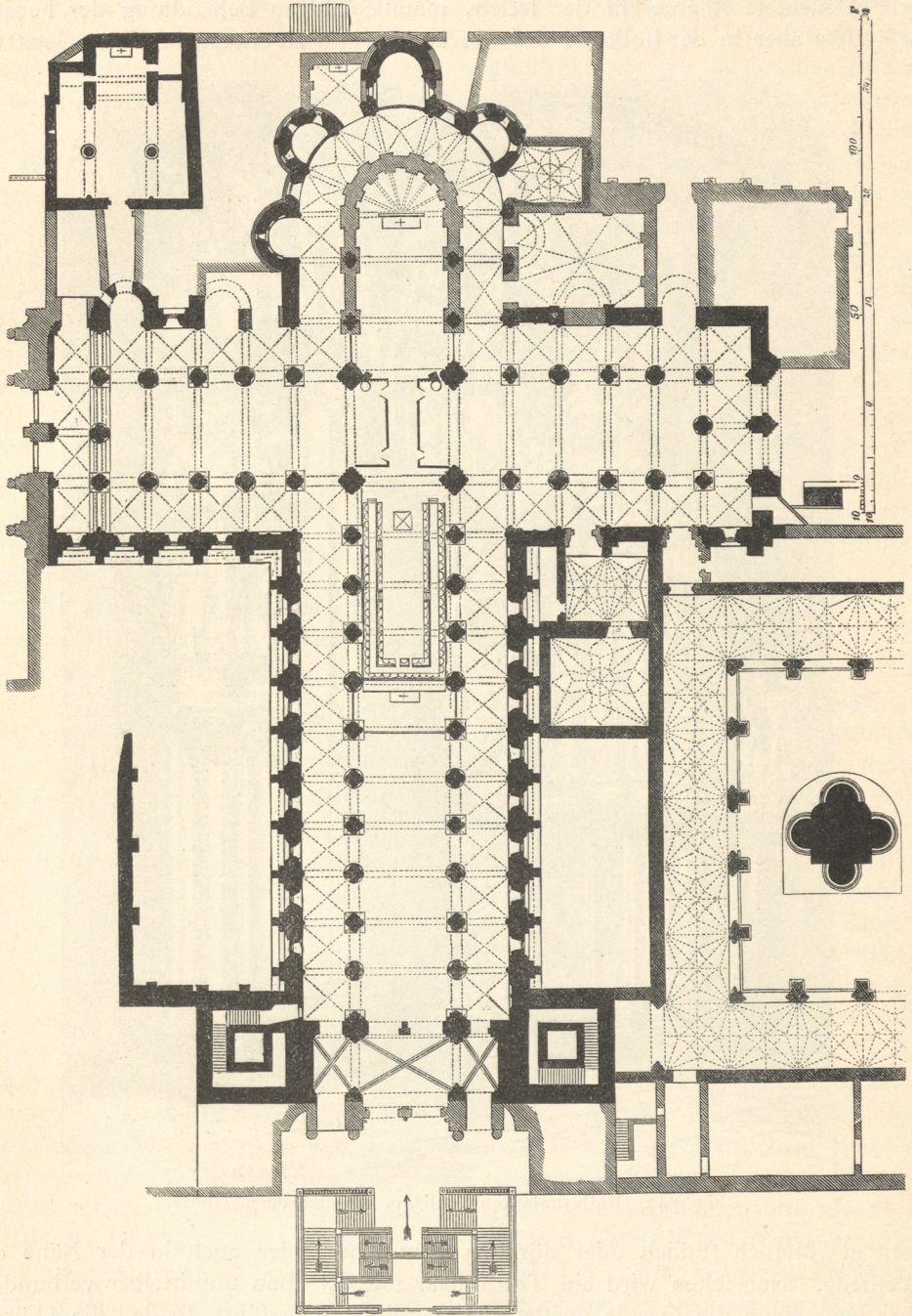
Fig. 543. Grundrifs der Kathedrale von Santiago de Compostella.
