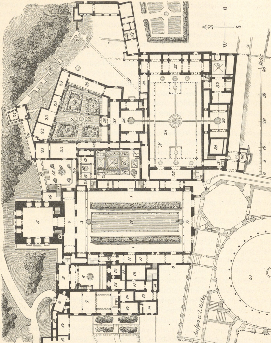
Fig. 383. Alhambra. Grundriss.
