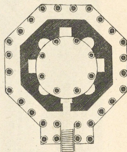
Fig. 311. Grundriss des fog. Juppiter-tempels zu Spalato.
