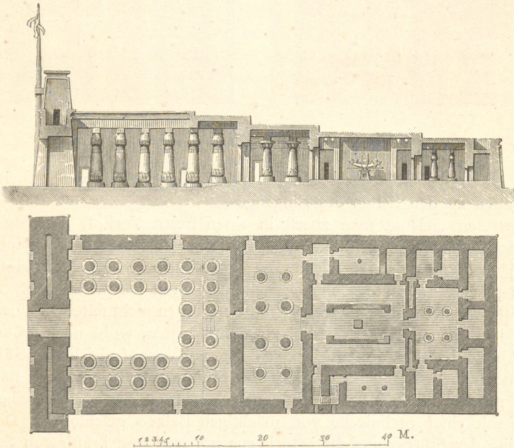
Fig. 12. Tempel des Chons zu Karnak (Längendurchschnitt und Grundrifs).
