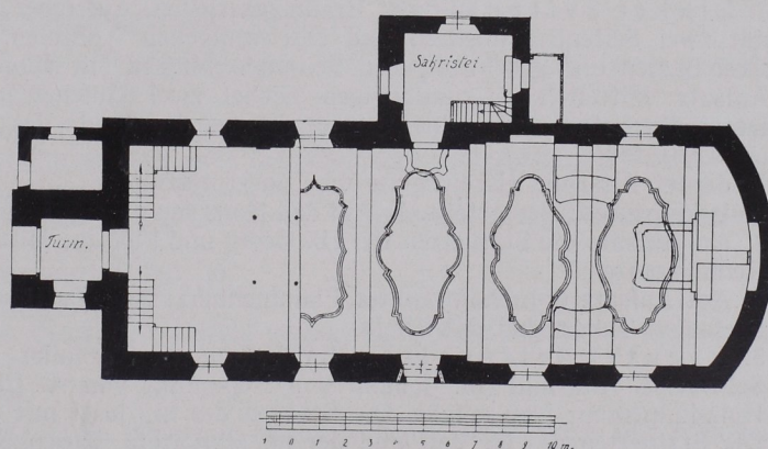
Abb. 240 St. Koloman, Pfarrkirche, Grundriß (S. 240).
