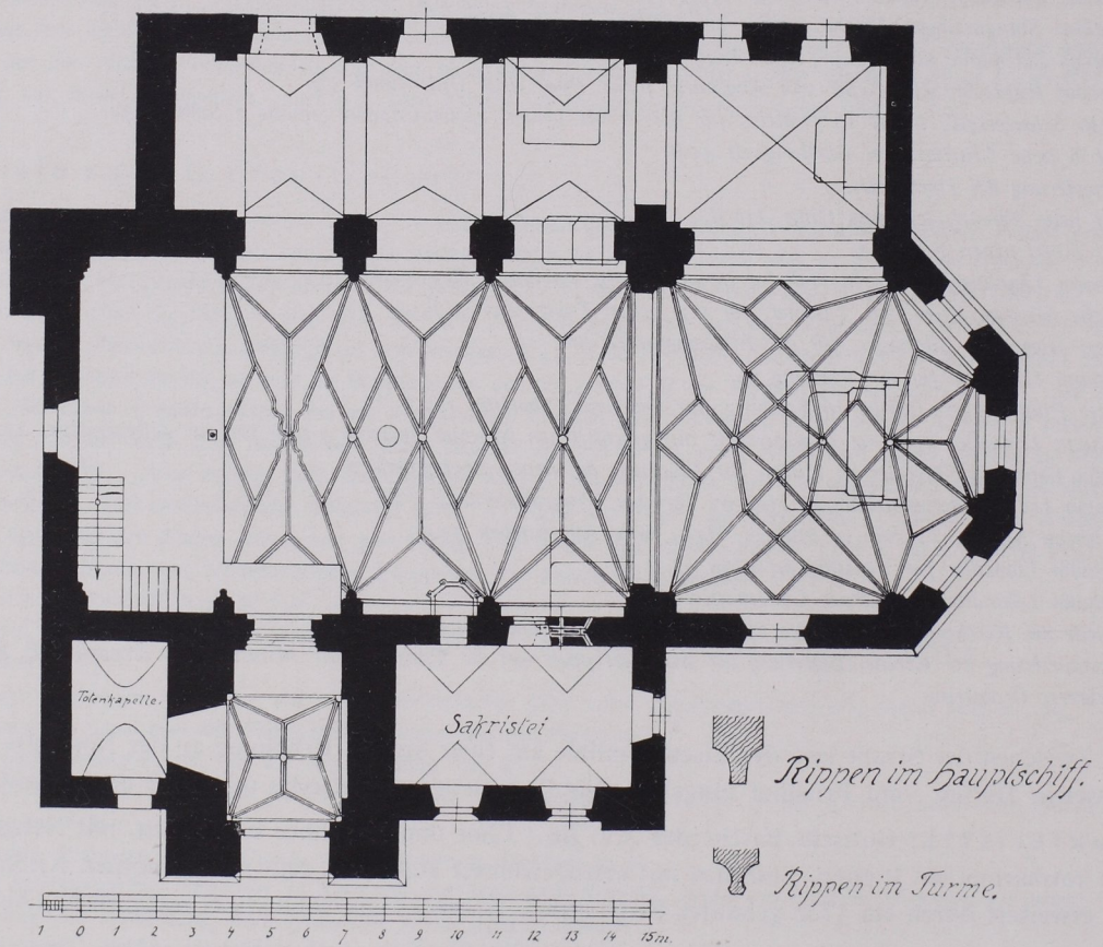
Abb. 208 Puch, Filialkirche, Grundriß und Aufriß 1:200 (S. 215).
