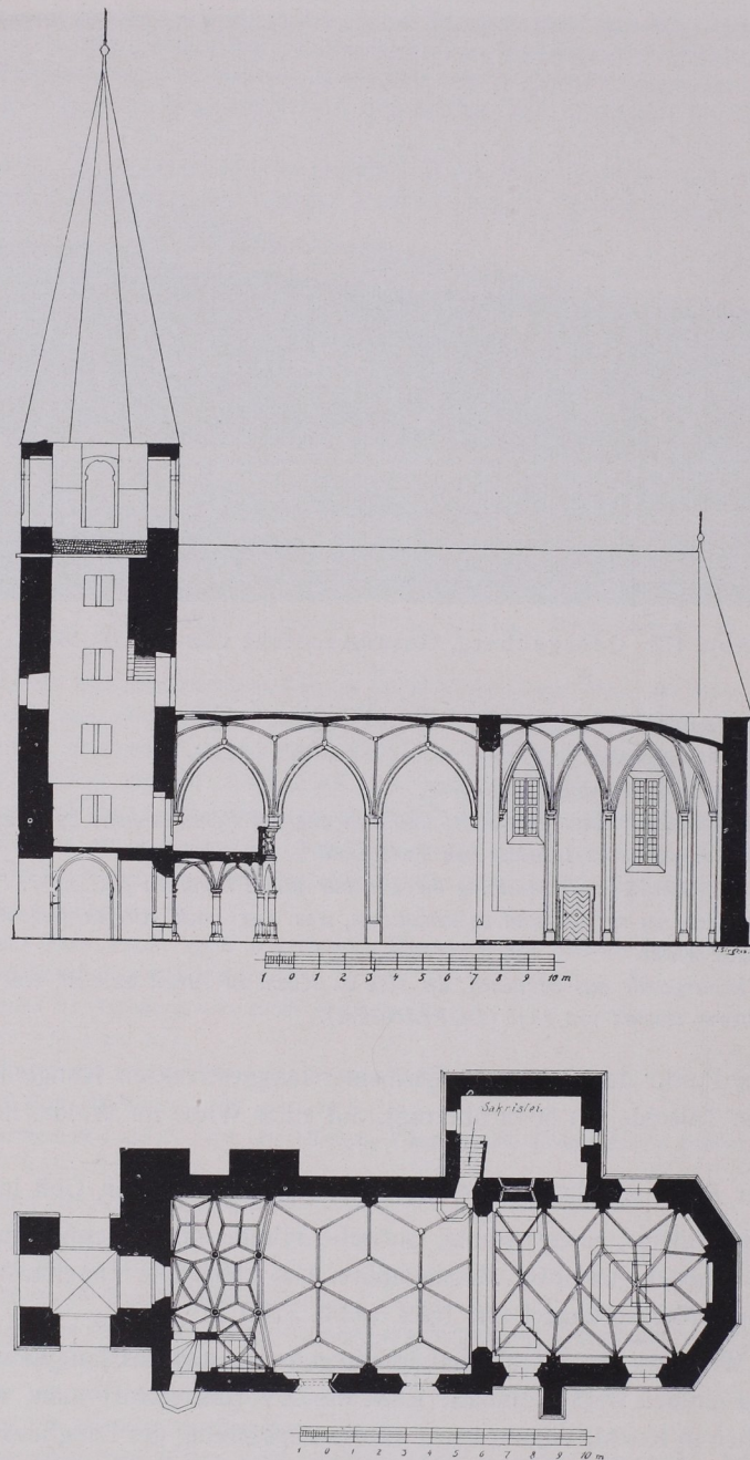
Abb. 178 Georgenberg, Grundriß und Längenschnitt 1:300 (S. 185).
