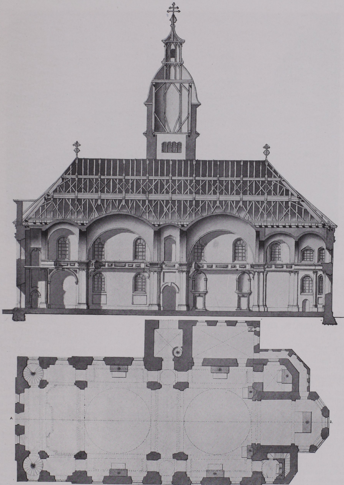
Abb. 79 Hallein, Pfarrkirche, Grundriß und Längenschnitt. Original von Simon Weibhauser, 1794, im Landesregierungsarchiv in Salzburg (S. 94).
