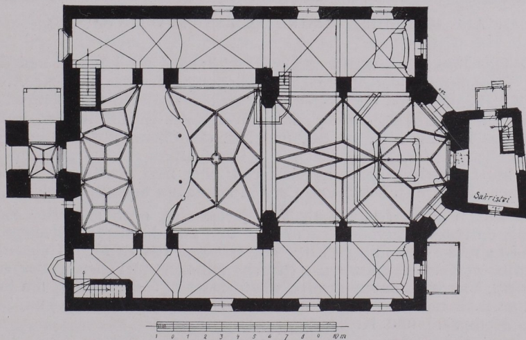
Abb. 65 Golling, Pfarrkirche, Grundriß und Längenschnitt 1: 300 (S. 72).
