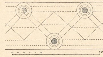
Grundriss und Schnitt vom Kreuzgang auf der Merveille in Mont Saint-Michel.
