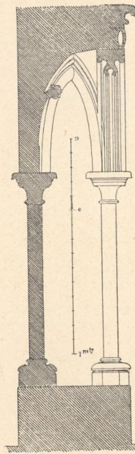
Grundriss und Schnitt vom Kreuzgang auf der Merveille in Mont Saint-Michel.
