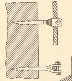
11. Befestigung der Wandleitung.
