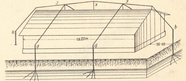
9. Anordnung der Blitzableitung, System Farady.
