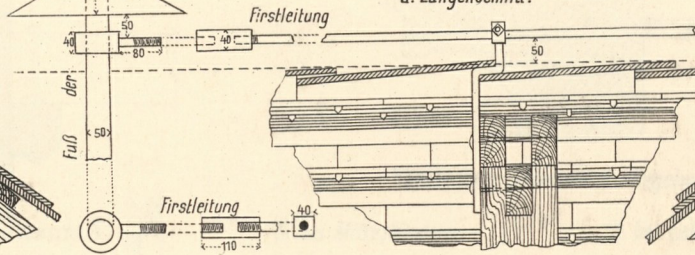
5. Befestigung der Firstleitung.
