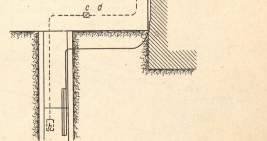
17. Schema zur Untersuchung von Blitzableitern im Profil.
