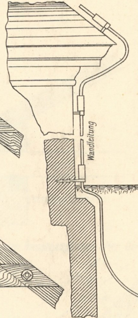
6. Befestigung der Dachleitung.
