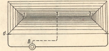
16. bei 3 Auffangstangen.
