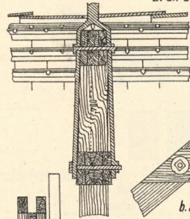
3. Befestigung der Auffangstange.
