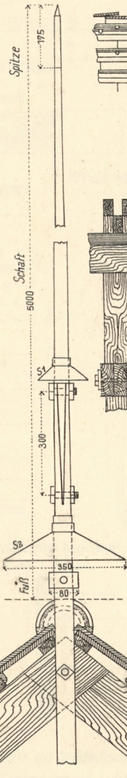
2. Auffangstange.
