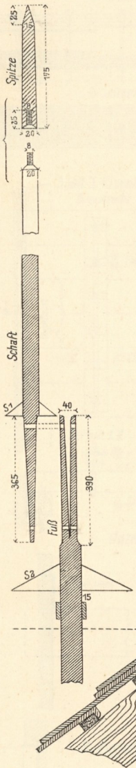
1. Detail der Auffangstange.
