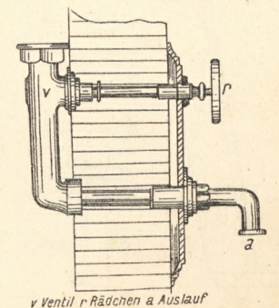
27. Frostsicherer Ventilhahn.
