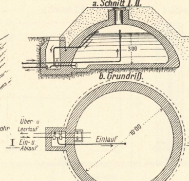
4. Wasser-Sammelbehälter.
