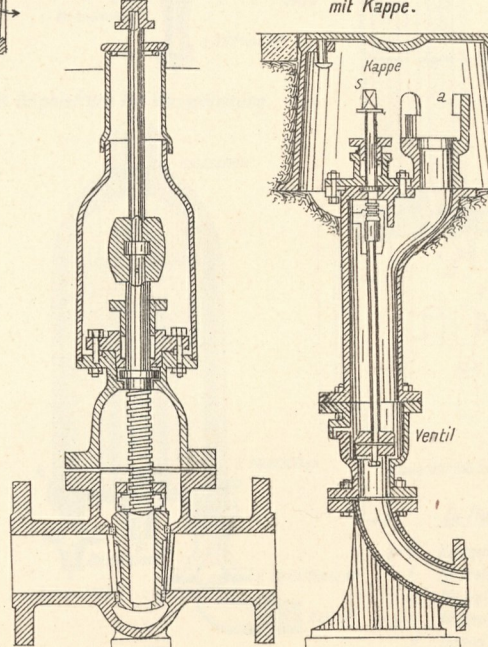
22. Schieberventil für Leitungen über 50mm Lichtweite.
