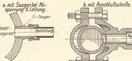
9. Anbohrung des Hausleitungsrohres.
