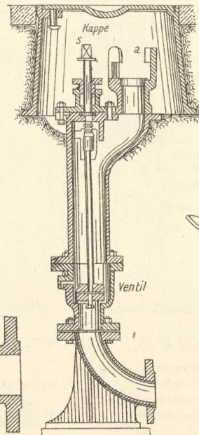
23. Hydrant mit Kappe.
