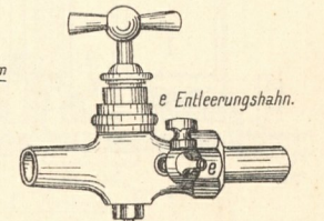
27. Frostsicherer Ventilhahn.
