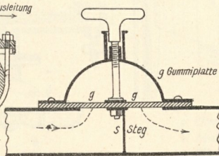
14. Gummihahn.
