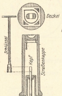
8. Ventil zum Absperrn d. Hausleitung.
