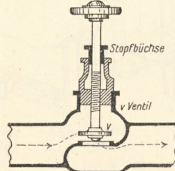
15. Ventilhahn.
