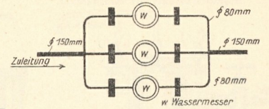
7. Wassermesseraordnung mit Rückschlagventil.
