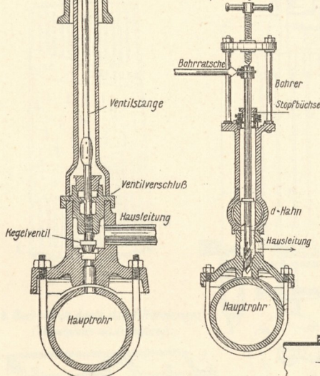
10. Anbohrung der Hauptleitung unter Druck.
