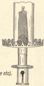
50. Zwergbrenner.
