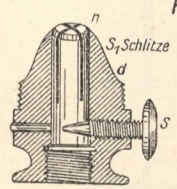
76. Schlitzdüse.
