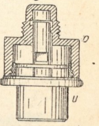
78. Behl'scher Konsumregler.
