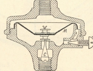
77. Membranregler.
