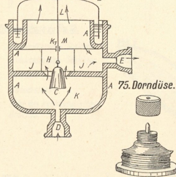
74. Gasdruckregulator. Bleiplatten.
