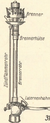
24. Laternenhahn mit Zündflamme.
