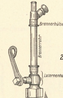
30. Einloch- brenner.
