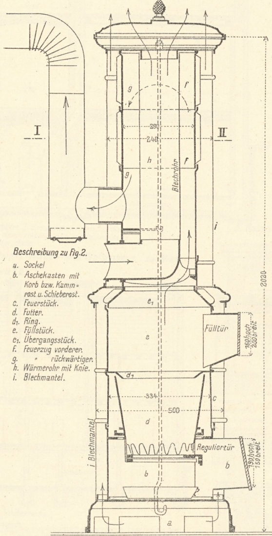
2. Normalkasernofen „Imperial“ a. Ansicht u. Vertikalschnitt.
