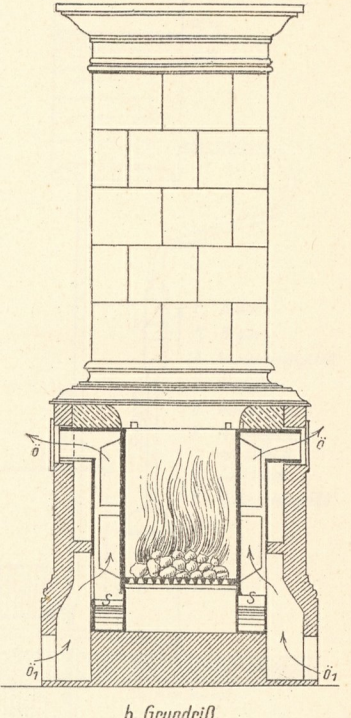
5. Kachelofen mit Heizmultiplikator. Patent Gasseleder und Niemecek.
