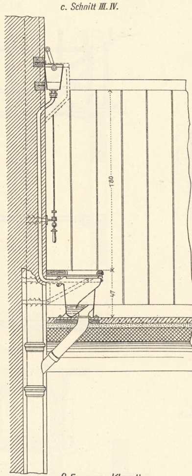
9. Fayence-Klosett, mit lackiertem Rückenreservoir aus Eisen.
