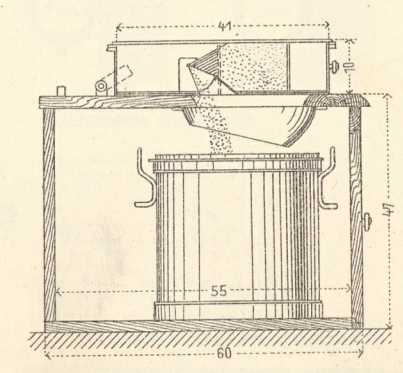
11. Torfmullstreuapparat, mit Beckelstrommagazin von W. Brückner.
