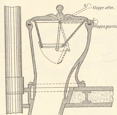
10. Abortanlage mit Torfmullstreuung. (Torfmullklosett).
