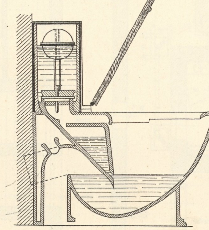
9. Fayence-Klosett, mit lackiertem Rückenreservoir aus Eisen.
