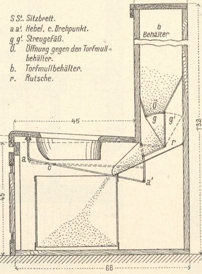
10. Abortanlage mit Torfmullstreuung. (Torfmullklosett).
