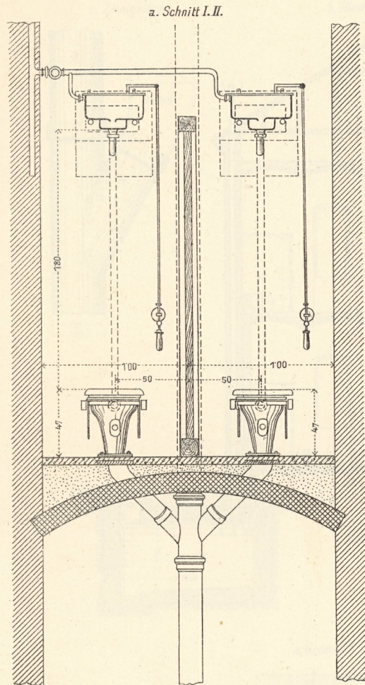
1. Freistehendes Klosett mit Hochhängspülkasten, gußeiserner „Danubia“-Schale und Niagara-Spülkasten.
