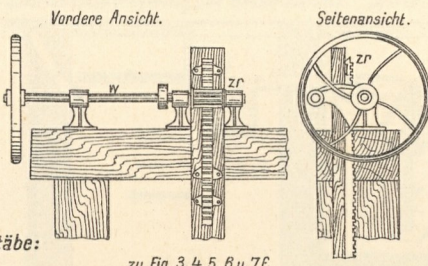
f. Detail der Aufzugvorrichtung.
