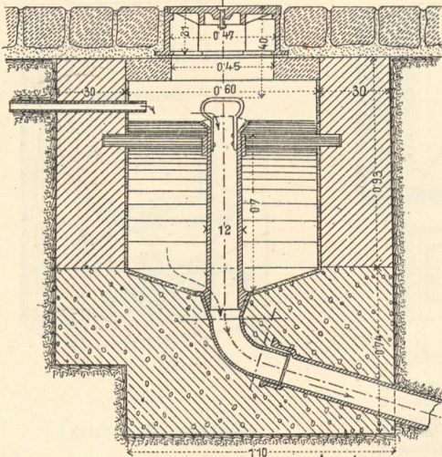
5. Schiammfang für Dachabfallrohre.
