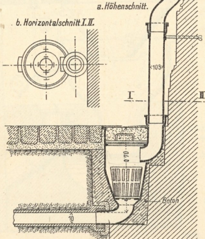
5. Schiammfang für Dachabfallrohre.
