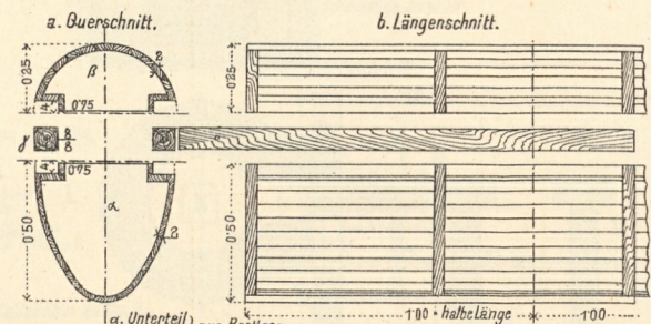
6. Holzene Form für die Ausführung von Betonkanälen.
