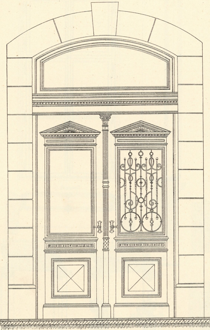
a. Ansicht.
