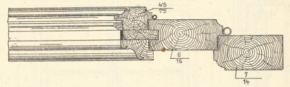
f. Schnitt durch die Mittelfrieze.
