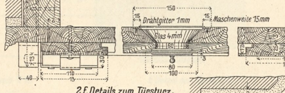
2f. Details zum Türsturz.
