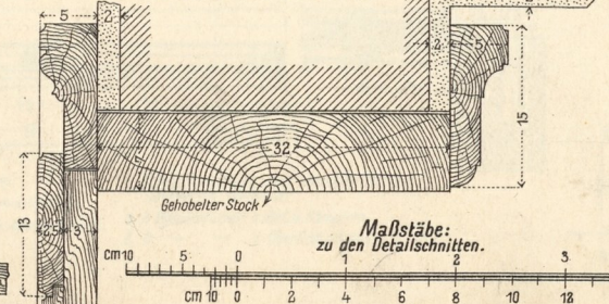
2f. Details zum Türsturz.
