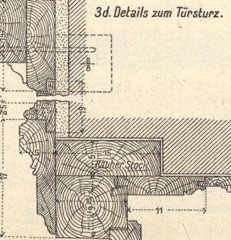
3d. Details zum Türsturz.
