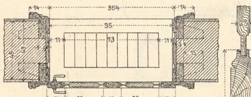
1d. Details zum Höhschnitt.
