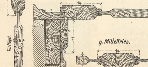
1f. Details zum Grundriß.
