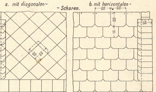
mit Schuppenschiefer.
