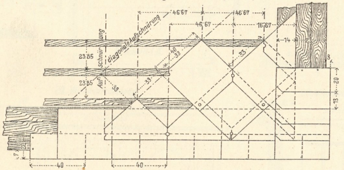
6. Deutsche einfache Deckung mit Quadratsteinen.
