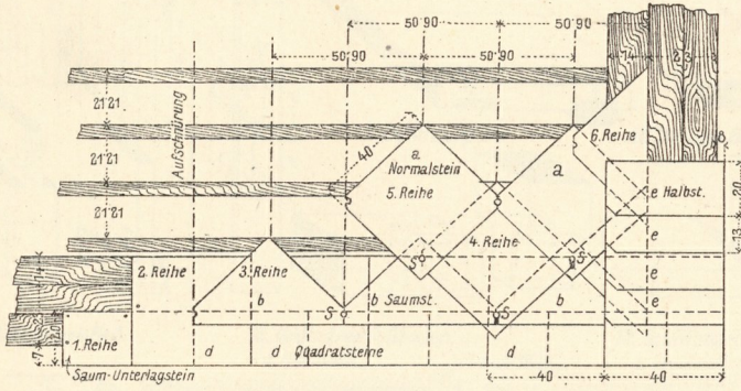
1a. Normalstein. 1b. Saumstein. 1c. Saumunterlagsstein. 1d. Quadratstein.
