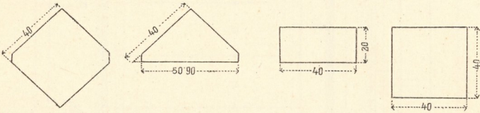
5. Französische Eindeckung ohne überhängende Spitzen.
