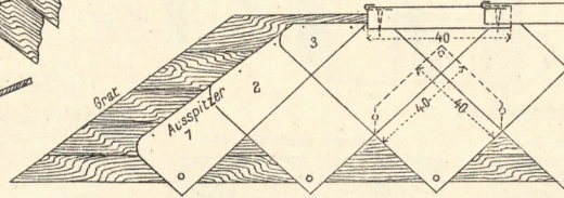
3b. Hohlstein.
