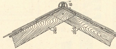
3a. Befestigung der First- u. Grathohlsteine mit Klammern.
