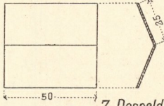
7. Doppeldeckung mit Quadratsteinen.
