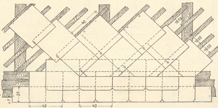
6. Deutsche einfache Deckung mit Quadratsteinen.
