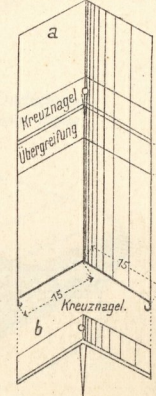
14. First- u. Gradblech.
