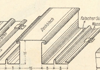
B. mit falschem Stehfalz.
