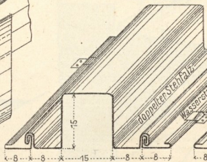
A. mit Stehfalz.
