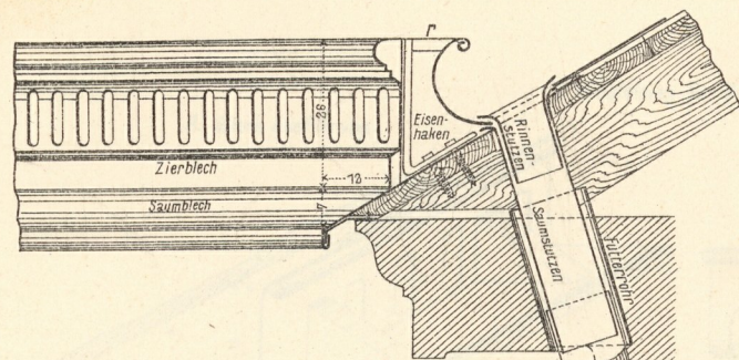
2. Abfallrohr mit eisernem Schutzständer.
