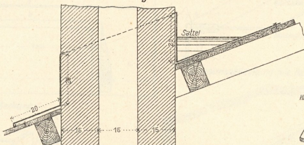
13. Brand- und Feuermauereindeckung.
