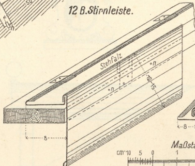
12 B. Stirnleiste.
