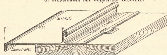
10. Giebelsaum mit falschem Stehfalz.
