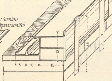
C. Feuermauer.
