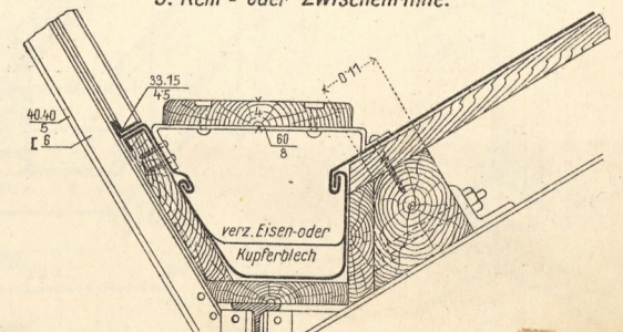
9. Kehl- oder Zwischenrinne.
