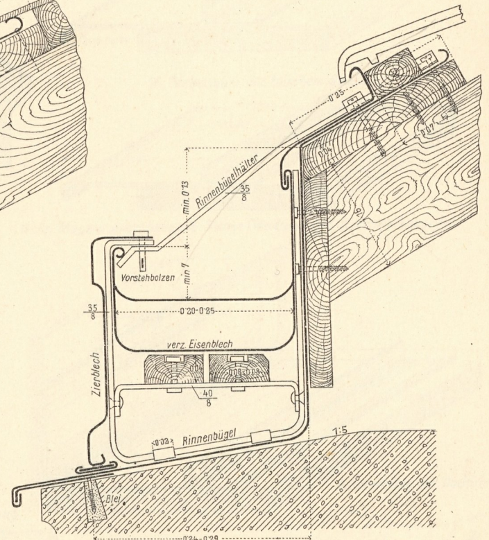
8. Kehlrinne bei Sheddächern.
