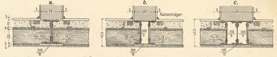
7. Decke mit Unterzügen und Säulen aus Schmiedeeisen.
