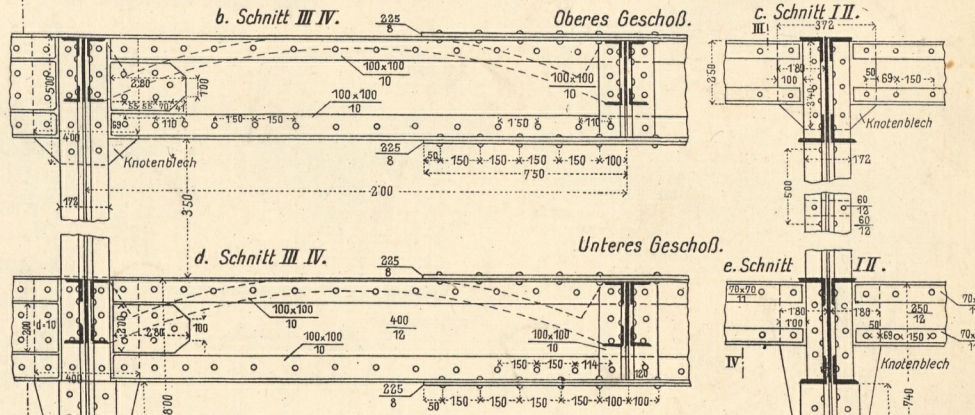
7. Decke mit Unterzügen und Säulen aus Schmiedeeisen.
