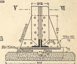
F. Sockel.
