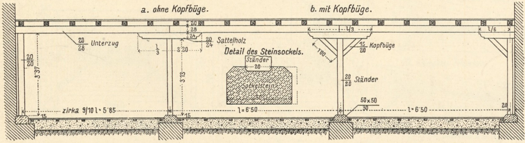
4. Tramdecke mit hölzernen Unterzügen und Ständern für zwei Geschoße.
