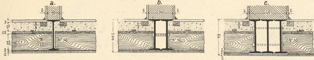
1. Gewalzte Mauerträger.
