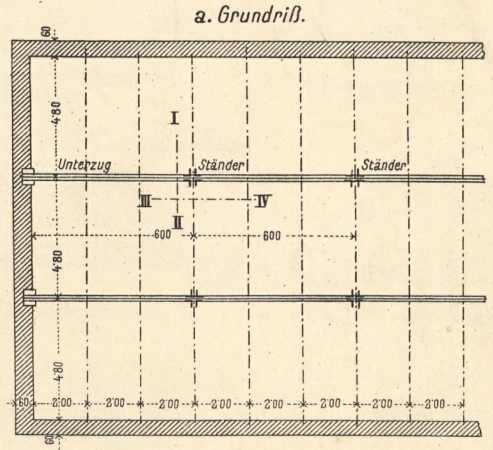
8. Eisenbetonsäule.
