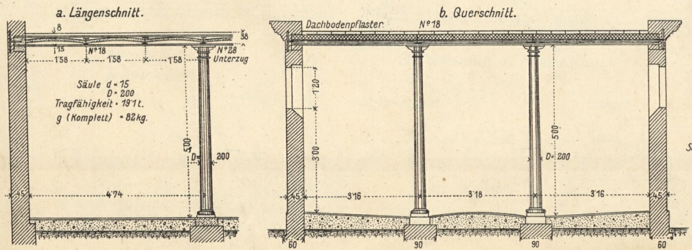
6. Gewölbsdecke zwischen I Trägern mit Unterzügen und gußeisernen Säulen, z.B. für ein Stallgebäude.
