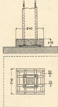
8. Eisenbetonsäule.
