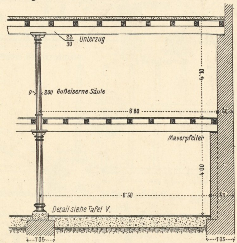
6. Gewölbsdecke zwischen I Trägern mit Unterzügen und gußeisernen Säulen, z.B. für ein Stallgebäude.
