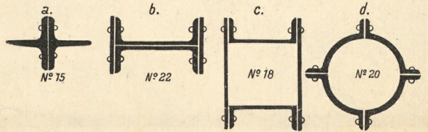
9. Querschnitte von schmiedeeisernen Ständern.
