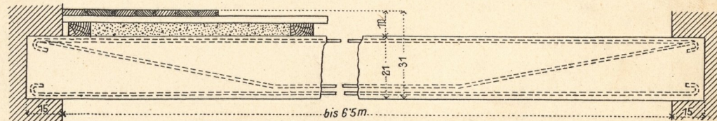
Lagerung der Siegartbalken.
