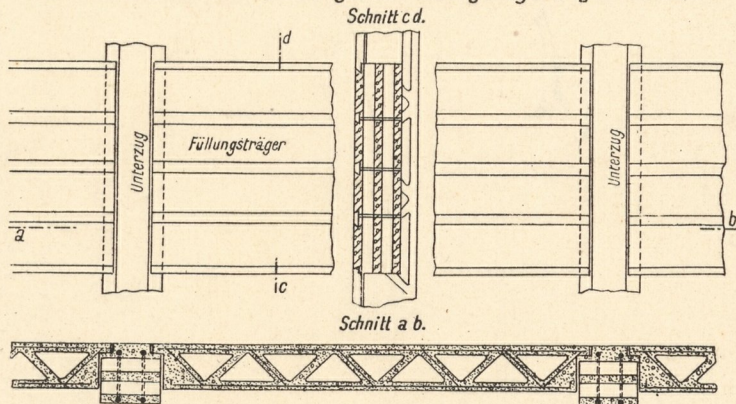
Bogenbalkendecke, System Thrul.
