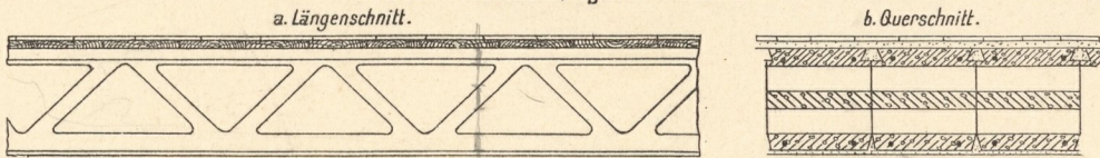
3. Eisenbetondecke mit Unterzügen und Füllungsträgern, Syst. Visintini.
