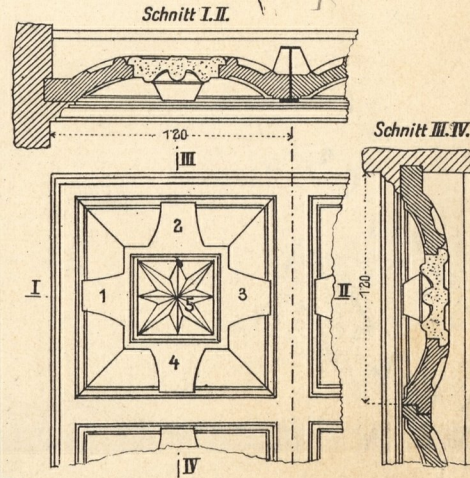
13. Mit 5 Kassettenteilen (1 bis 5).
