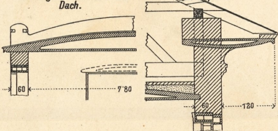
8. Die Bogenbalken als Gesimshängplatte.
