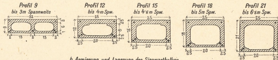
b. Armierung und Lagerung der Siegartbalken.
