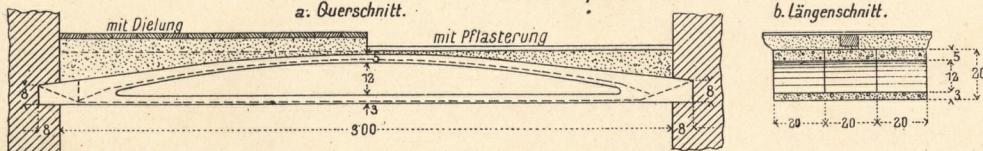
6. Für 6m Spannweite.
