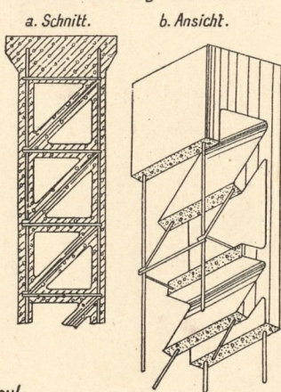
4. Betonsäule, Syst. Visintini.
