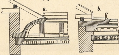
11. Hauptgesimse aus Eisenbeton.
