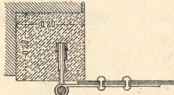
7. Eiserne Tür mit Winkeleisenrahmen.
