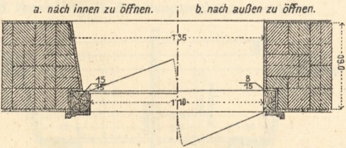
4. Spalettür mit hölzernem Stock.
