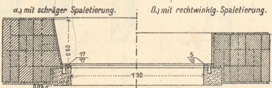
4. Spalettür mit hölzernem Stock.
