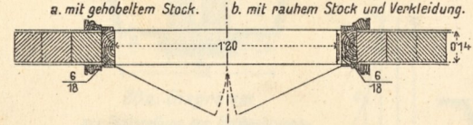
5. Futtertür bei 15 oder 30cm breitem Stock.
