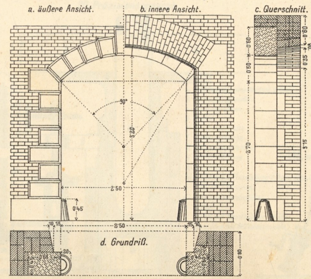
8. Tor mit Quaderverkleidung.
