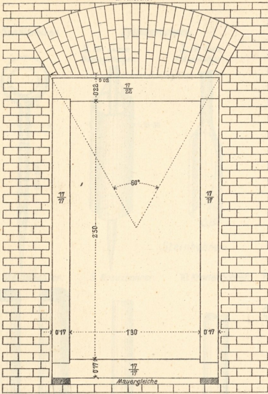
1. Spalettür mit steinernem Stock in der Mauerflucht. a. Ansicht.
