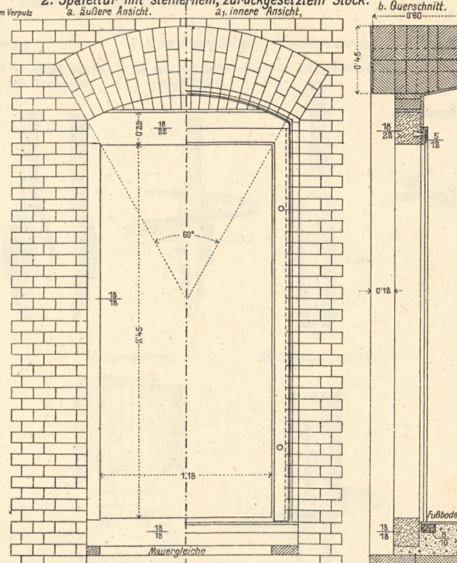
2. Spalettür mit steinernem, zurückgesetztem Stock. a. äußere Ansicht. a1. innere Ansicht.
