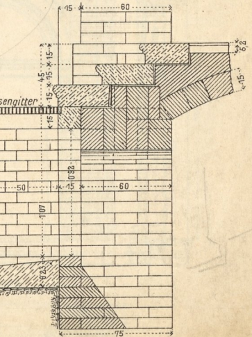
14. Kellerfenster mit Lichtsacht, unter einem Eingange.
