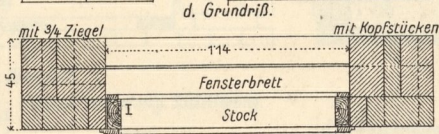
11. Fenster mit steinernem Stock.
