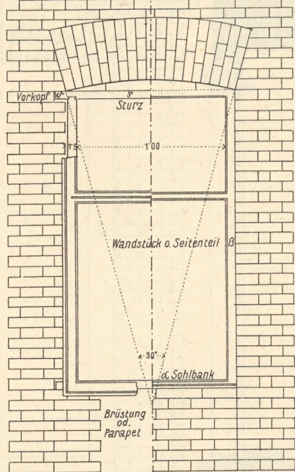
6. Nach außen aufgehendes Fenster.
