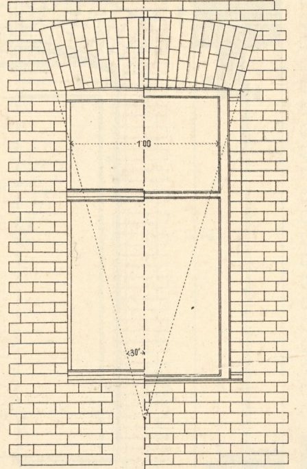
7. Zurückgesetztes, nach innen aufgehendes Fenster.
