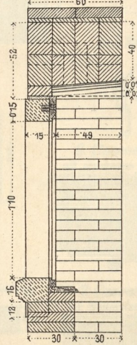
b. Querschnitt.
