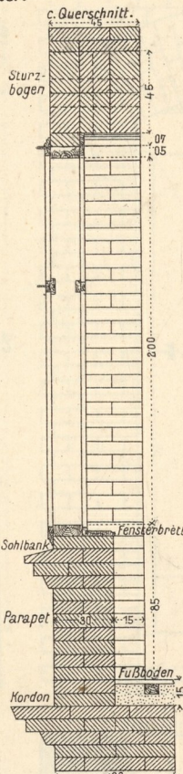
6e. Detail bei I.
