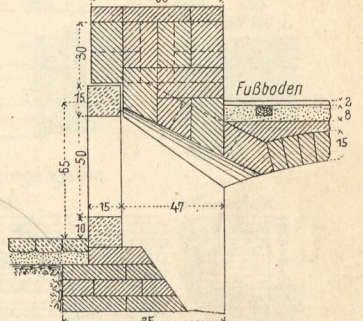
14. Kellerfenster mit Lichtsacht, unter einem Eingange.
