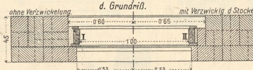
12. Kellerfenster mit Lichtsacht.
