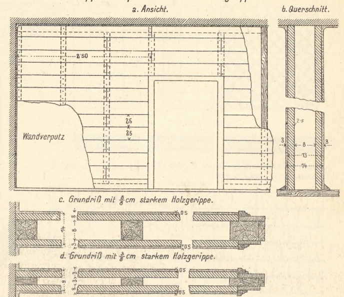
4. Einfache Gipsdielenwände zwischen Holzgerippe oder zwischen eisernen Trägern.
