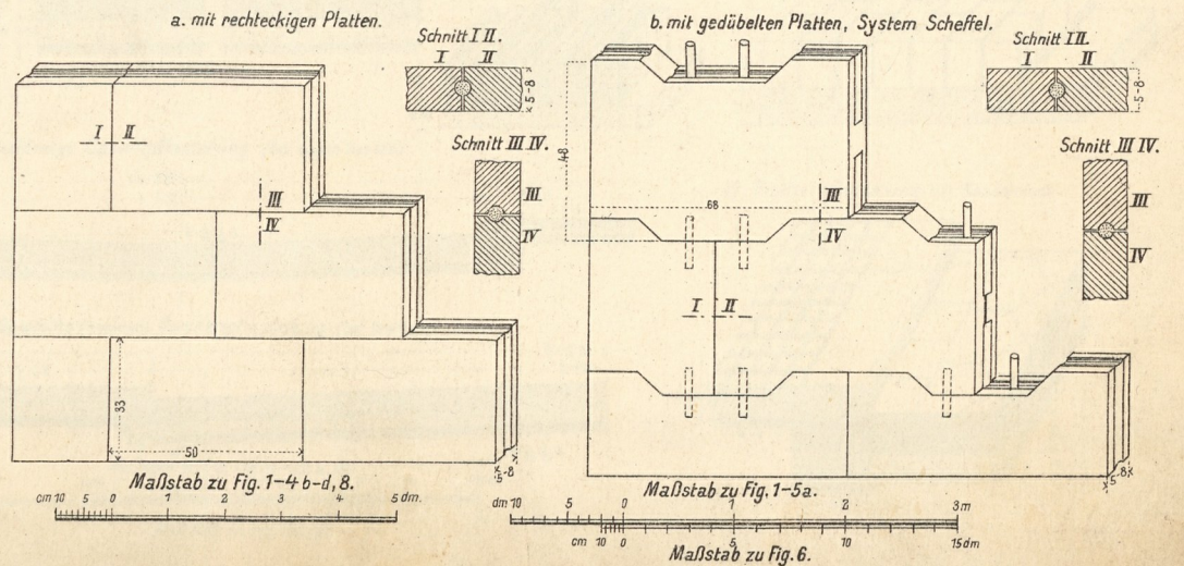
10. Gipschlackenwände.
