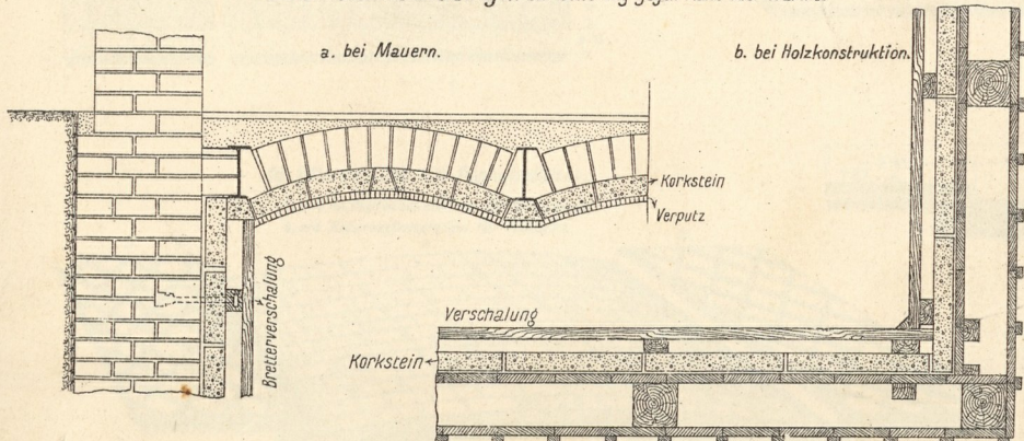
6. Korksteinverkleidungen zur Isolierung gegen Kälte oder Wärme.
