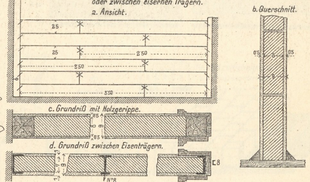
10. Gipschlackenwände.
