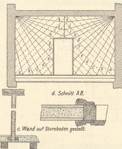
6. Korksteinverkleidungen zur Isolierung gegen Kälte oder Wärme.
