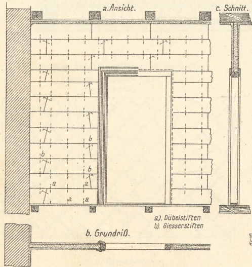
6. Korksteinverkleidungen zur Isolierung gegen Kälte oder Wärme.
