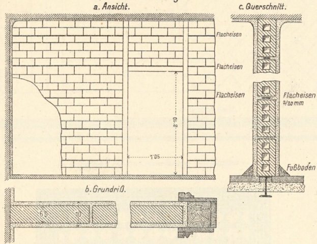
1. Scheidewand mit hochkantig gelegten, gewöhnlichen Ziegeln und Flacheisen-Einlagen.
