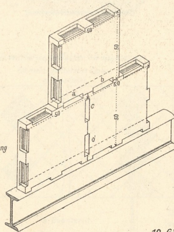
9. Skagliowände.
