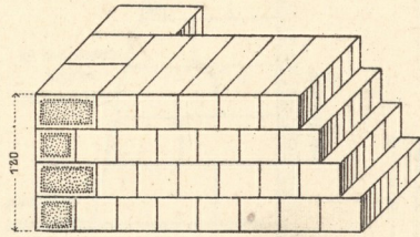
6. mit Läufern u. Bindern.
