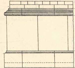
a. Ansicht.
