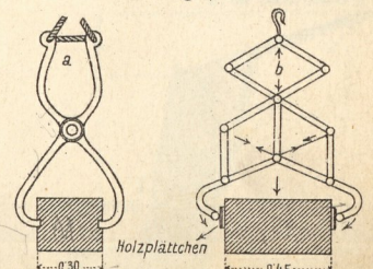
16. Zangen.
