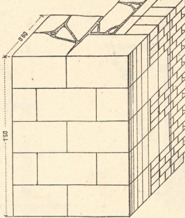
19. Stumpfwinkl. Eckarmierung m. Quadrern.
