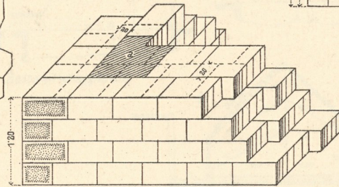
6. mit Läufern u. Bindern.
