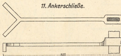
11. Ankerschleife.
