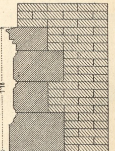
b. Profil.
