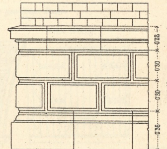
a. Ansicht.
