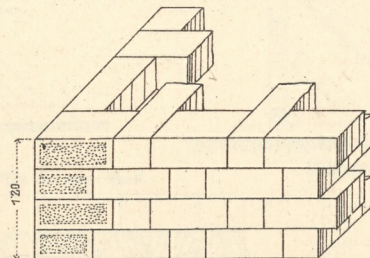
8. Quaderverkleidung m. Verankerung d. Stoßfugen.
