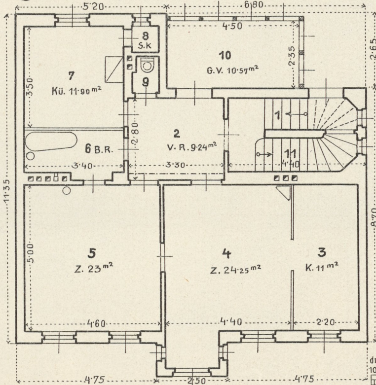
③ 121 m 2 M.B., 11.62 m 2 H.B., H.P. (1. St.)
