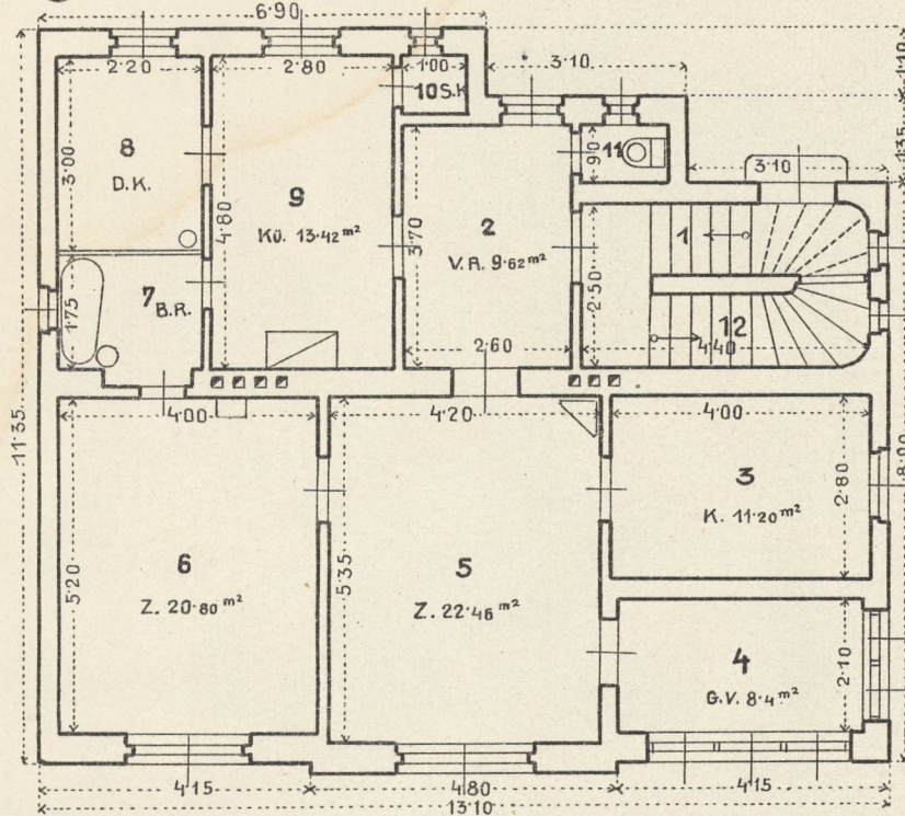
① 138.28 m 2 M.B., H.P. (1. St.)
