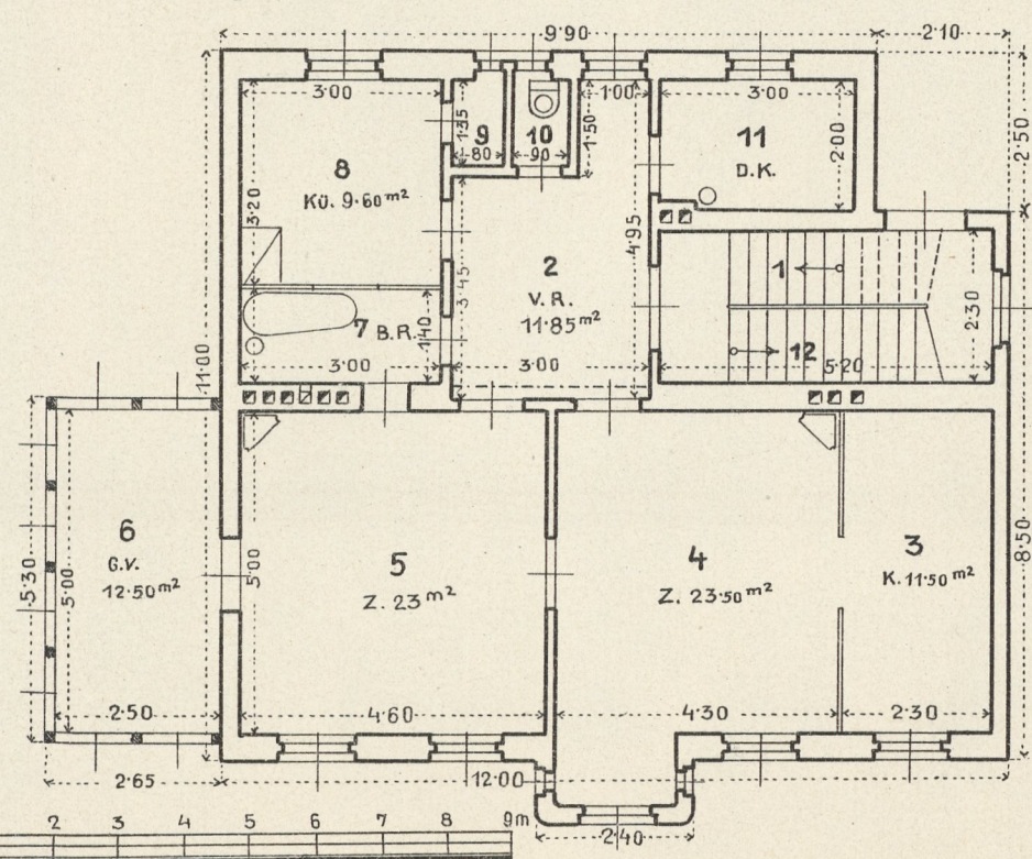
④ 129.15 m 2 M.B., 14 m 2 H.B., H.P. (1. St.)
