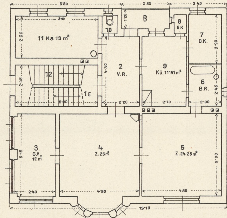
4. Zweigeschoßig für 2 Fam. mit je 2 Zim. Kab. Küche, Veranda u. s. w. 150 m 2 M.B.
