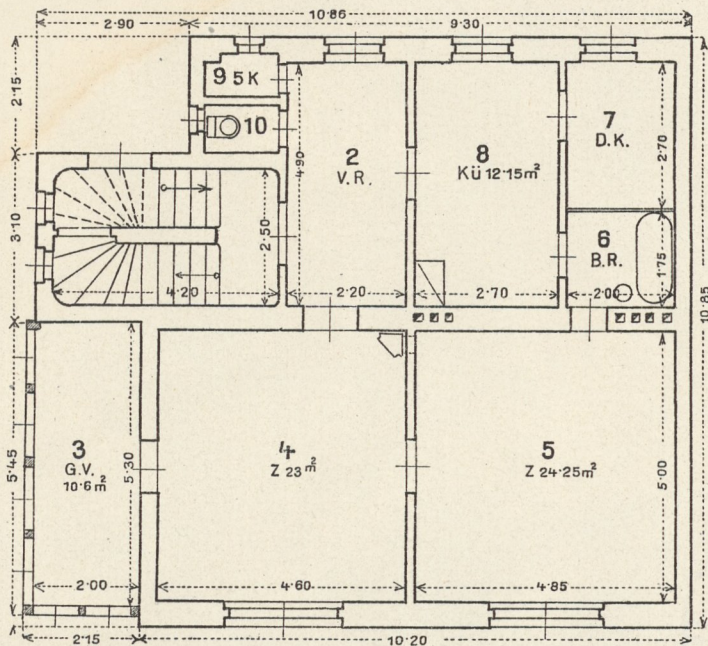
3. Zweigeschoßig für 2 Fam. mit je 2 Zim. Kab. Küche u. s. w. 143·77 m 2
