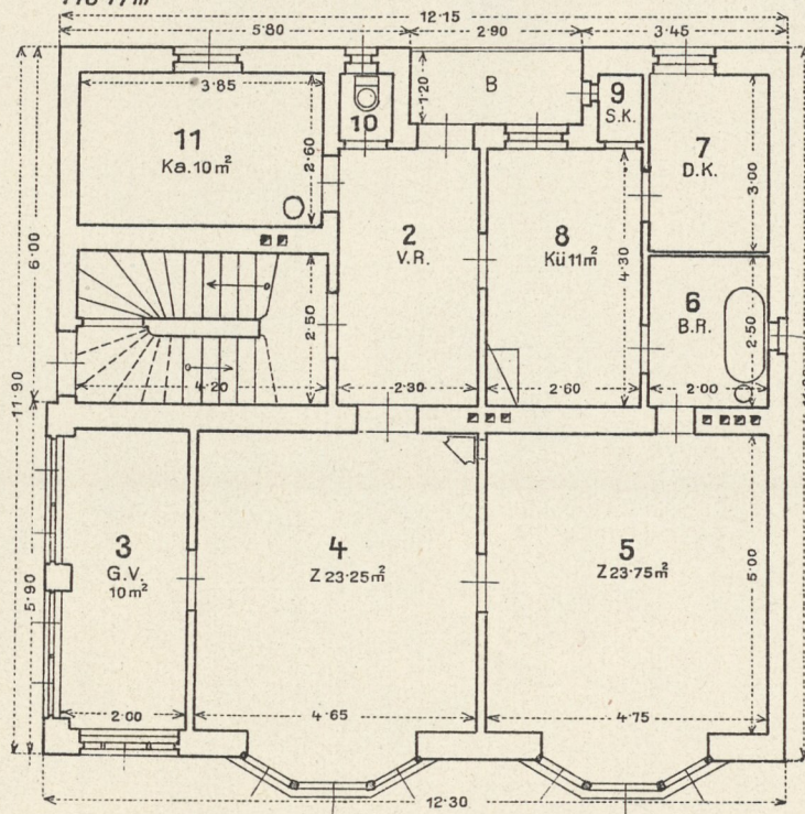
3. Zweigeschoßig für 2 Fam. mit je 2 Zim. Kab. Küche u. s. w. 143·77 m 2
