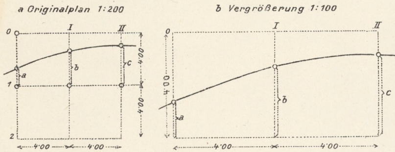
Fig.9. Vergrößern von Schichtenplänen mit Hilfe von Profillinien
