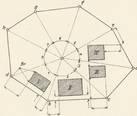
Fig.2 Aufnahme eines Grundkomplexes mit der Polarmethode
