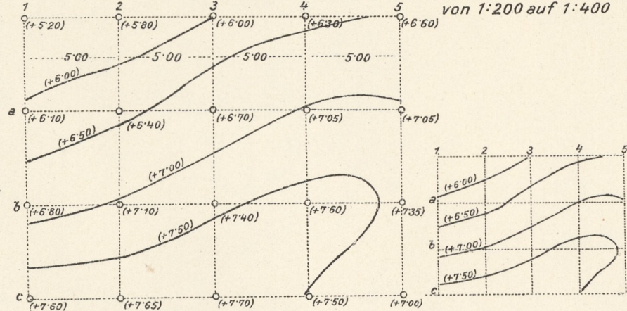
Fig.3 Terrainaufnahme mit der Netzmethode 1:200
