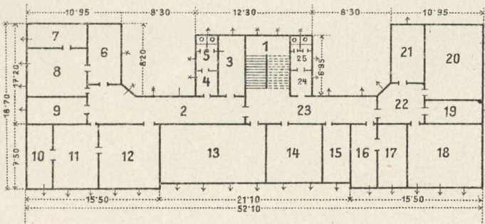
Fig. 9 Linearskizze 1/200
