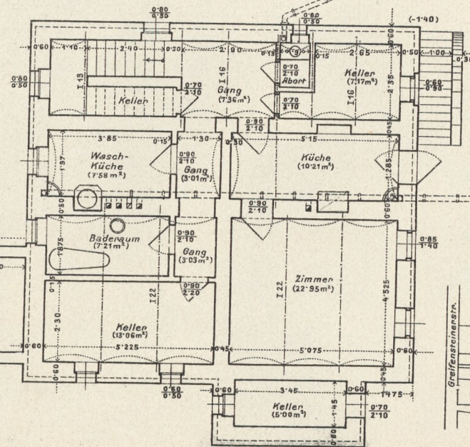
Fig. 2 Kellergeschoß 1/100
