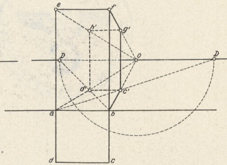
Schlagschatten Konstruktion.
