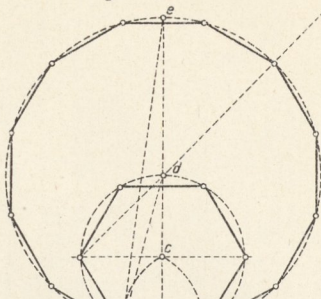
Fig.3. 6, 12 oder 24 Eck.
