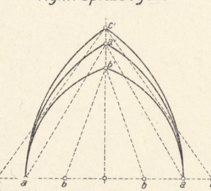
Gedrückte Spitzbögen.
