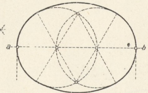
Fig.8. Ovale.
