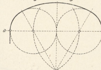
Fig.9. Korbbogen.
