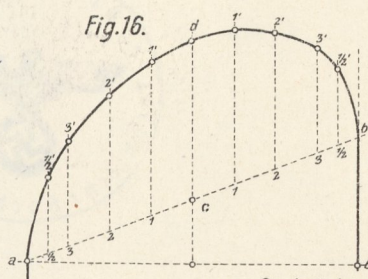
Gedrückte Spitzbögen.
