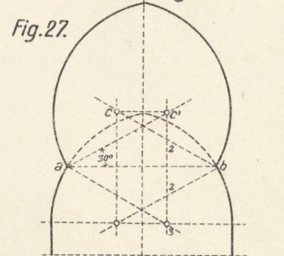
Hufeisenbögen.
