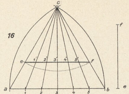
Graphische Reduktion von Maßstäben
