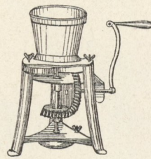
4. Farbmühle.
