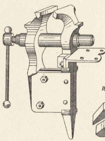
9. Schraubstock.
