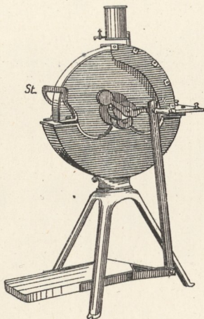
16. Schleifstein.
