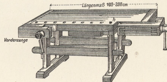
20. Hobelbank.
