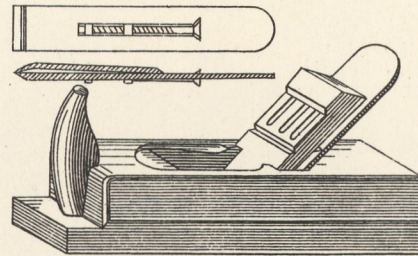
6. Kittfalzhobel.
