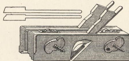
10. Nuthobel.
