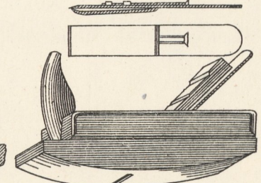
15. Schiffhobel.
