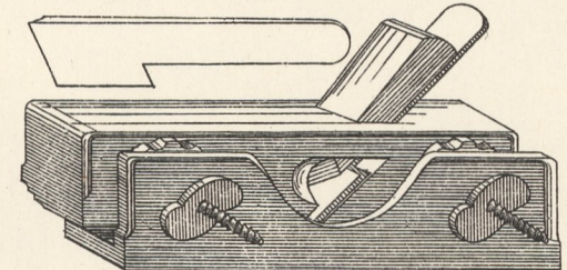
7. Plattbankhobel.
