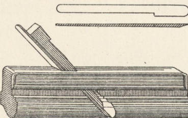
13. Hohlkehelhobel.
