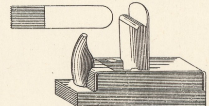
11. Zahnhobel.
