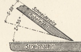
22. Schleifen der Hobeisen.
