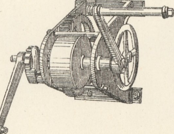
21. Sicherheits-Wandwinde Universal.
