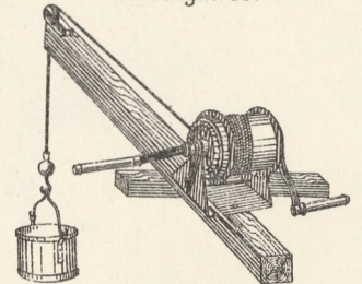
21. Sicherheits-Wandwinde Universal.
