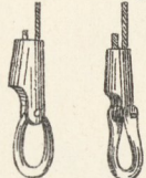
30. S-Haken mit Sicherheits-Verschlussscheibe.
