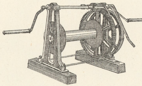
18. Aufzugwinde (Haspel) mit Leitrollen n-n'
