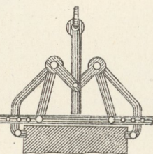
33. Kniehebel-Steinzange.
