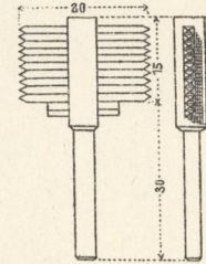
40. Schlageisen für harte-Steine b. weiche-Steine.
