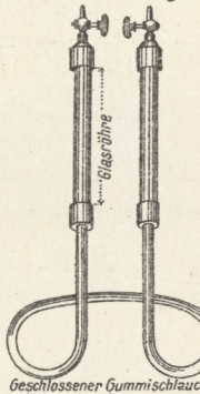
18. Schlauchwage.
