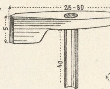
31. Bossierhacke.
