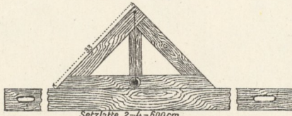
20. Setzlibelle.
