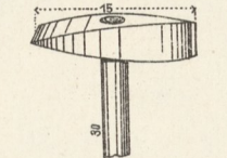
13. Ziegelputzhammer.
