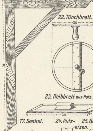
21. Rechter Winkel, aus Holz.
