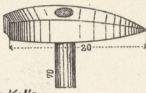
3. Gezähnte Kelle.
