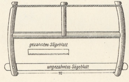
47. Steinhandsäge.
