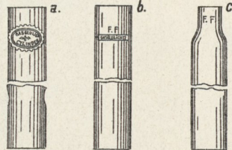
61. Jenaer Zylinder.
