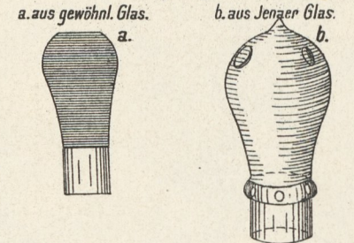
67. Glimmer- oder Marienglaszylinder für normale a.
