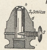
76. Schlitzdüse.
