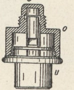
78. Behl'scher Konsumregler.
