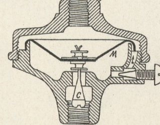
77. Membranregler.
